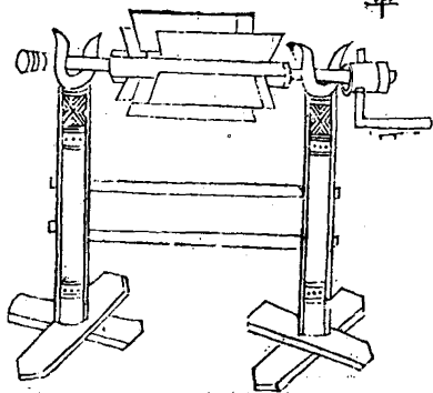
風扇車
