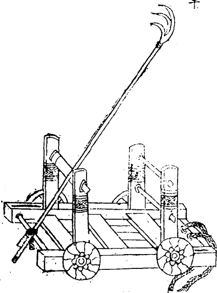
海車
